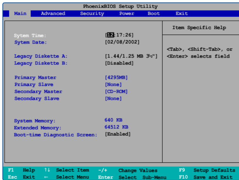
Gambar 76. Konfigurasi BIOS
